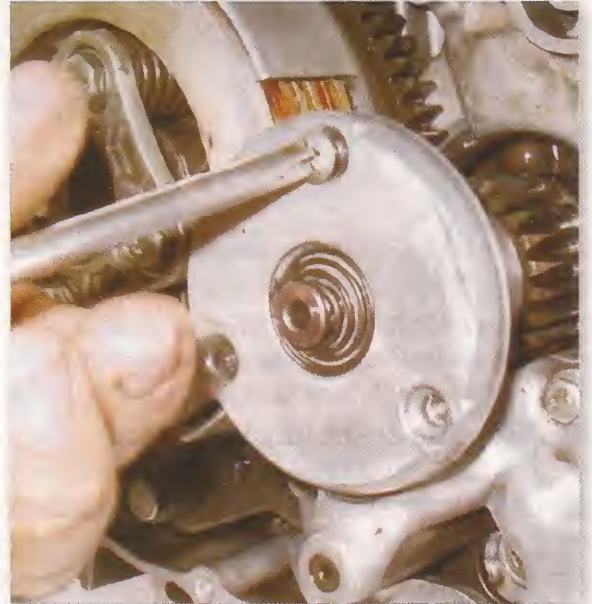
Destapando filtro centrífugo de aceite
